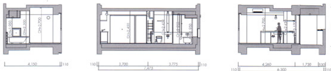
B2 / 断面図 (S=1/170)
